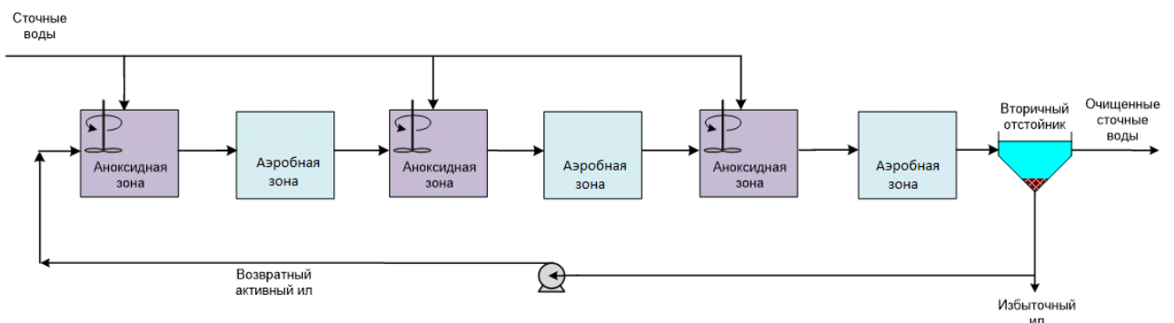
б) Ступенчатая нитри–денитрификация (могут использоваться 2 или 3 ступени с чередованием аноксидной и аэробной зон)
