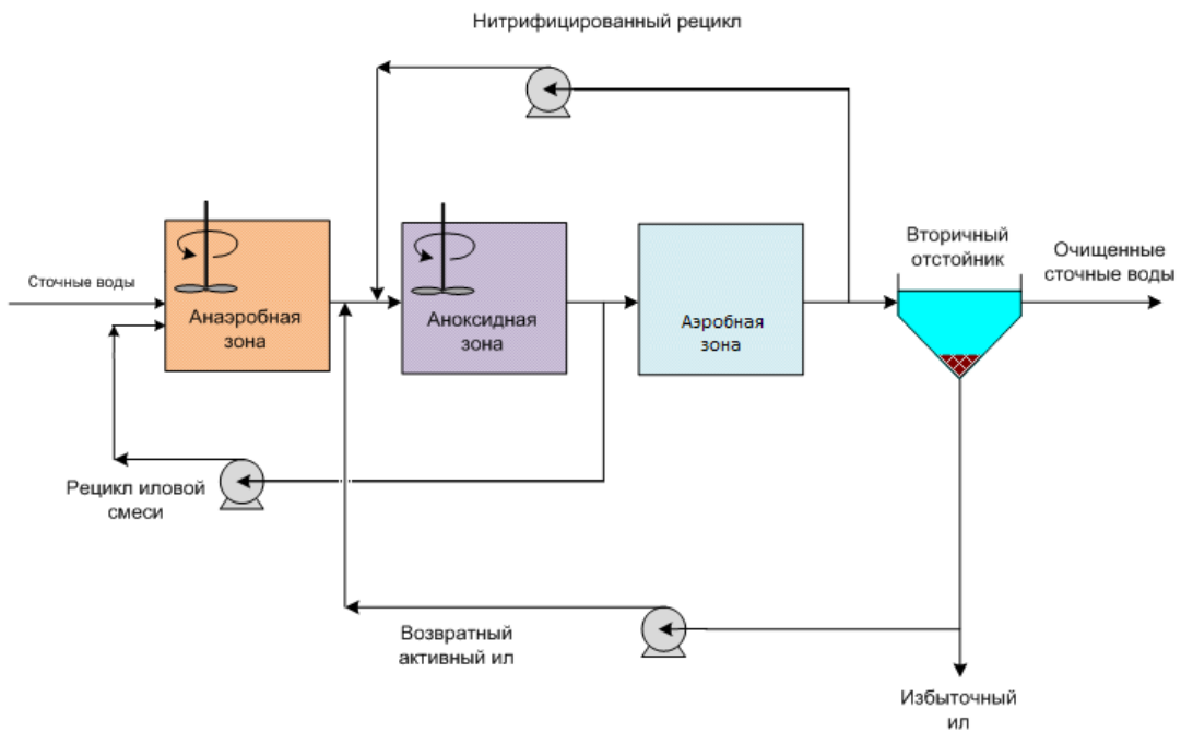
б) Процесс Кейптаунского университета (УСТ)
