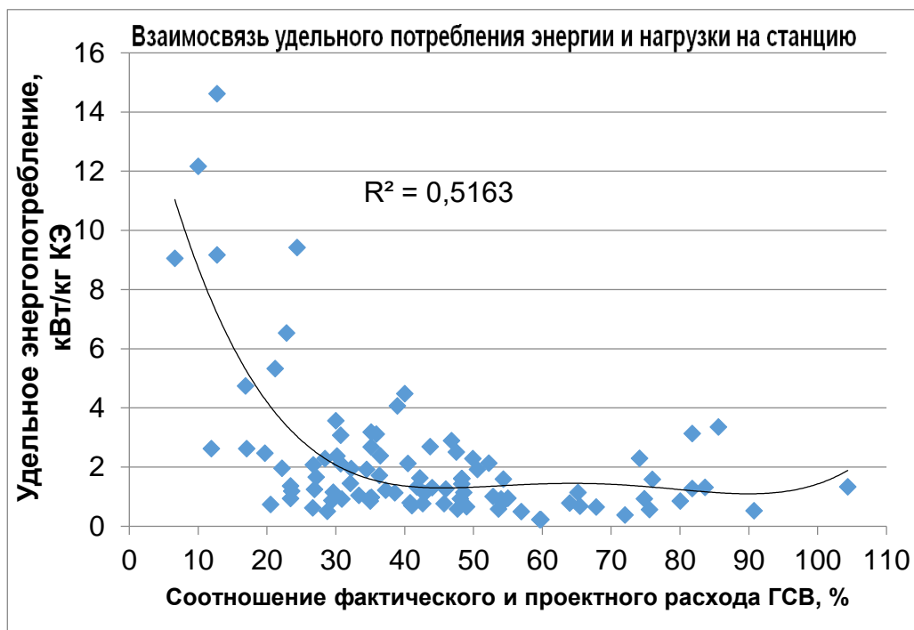
Рисунок 1.2 — Зависимость удельного энергопотребления от нагрузки на ОС ГСВ по сточным водам
