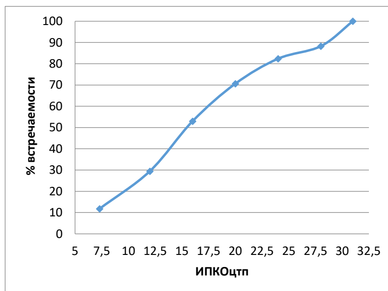
а) Для ОС ГСВ с ПП более 300 тыс. м 3 /сут
