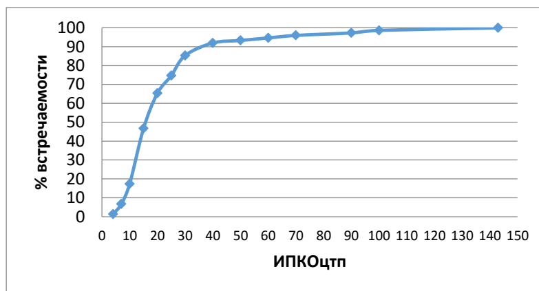
в) Для ОС ГСВ с ПП менее 100 тыс. м³/сут
